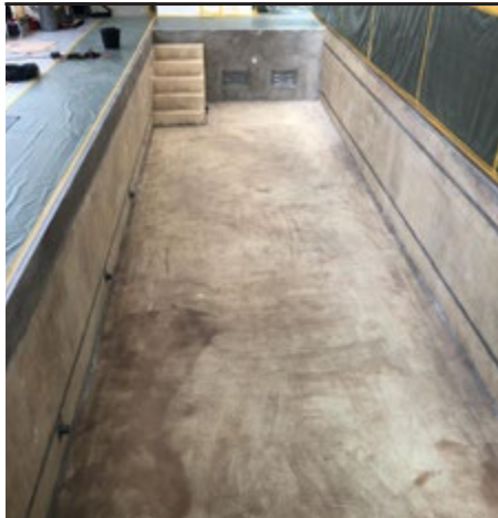
La superficie de hormigón lijada y con CP-Synthofloor BETA 8016 se espolvoreó con arena seca.
